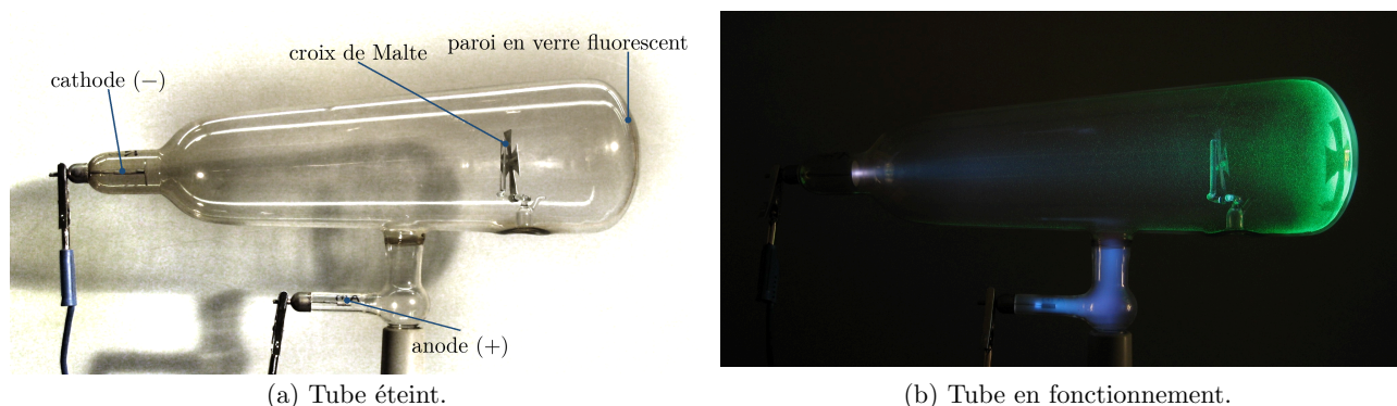
Fig. 1. – Tube de Crookes à croix de Malte. Les rayons issus de la cathode font fluorescer le verre en vert ; la croix les arrête et projette son ombre sur la paroi. Photos : D-Kuru/Wikimedia Commons.
